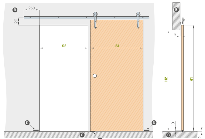
Skrzydło LOFT, dekor DĄB ST CPL, pochwyt okrągły, uchwyty skrzydła RETRO
