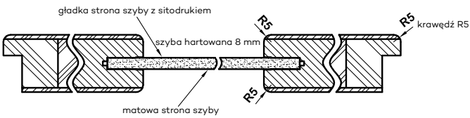
Przekrój poziomy drzwi VETRO A5, B5, D1
