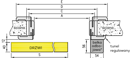
NT - przekrój poziomy (system lewy)
