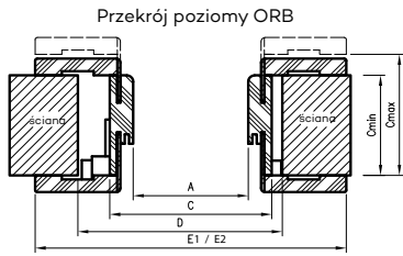
D - wymagana szerokość otworu w murze
