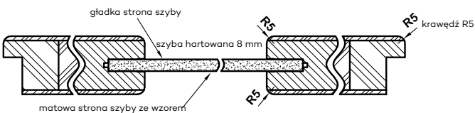
Przekrój poziomy drzwi VETRO A5, B5, D1
