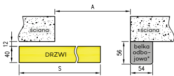
NS - przekrój poziomy (system lewy)
