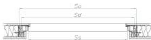
Drzwi HARMONY INVEST PRO otwierane do wewnątrz pod zabudowę panelową
