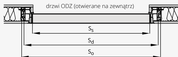
drzwi ODZ (otwierane na zewnątrz)
