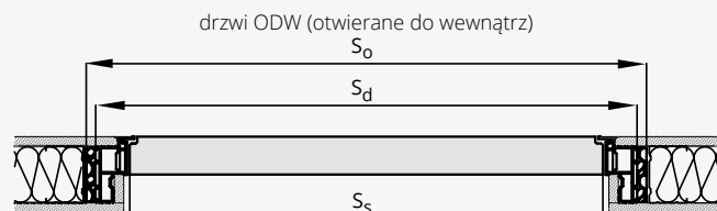
drzwi ODW (otwierane do wewnątrz)
